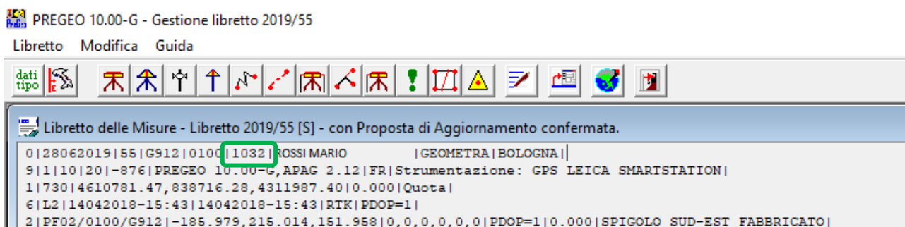
Figura 16 – Libretto delle misure corretto
